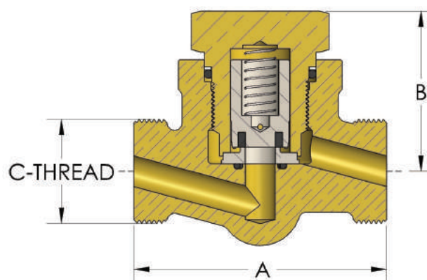
680 - Globe
