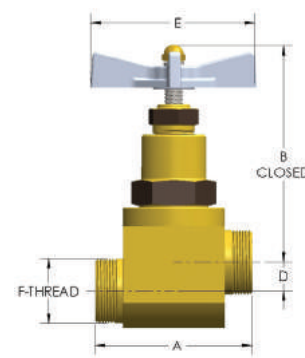
382 - Offset
